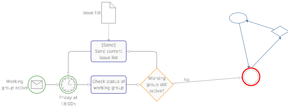
BPMN
